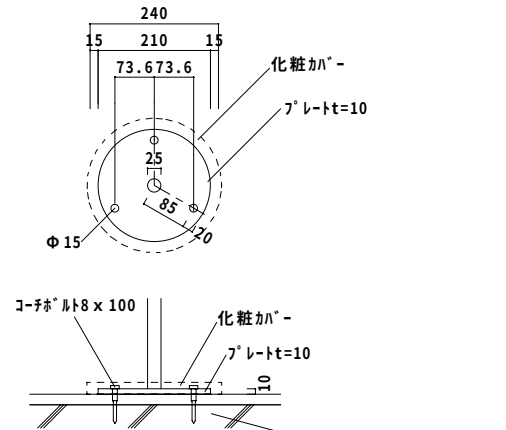
センターポール取り付け詳細図
