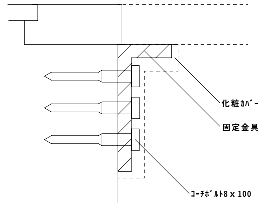
上部取付金具詳細図
