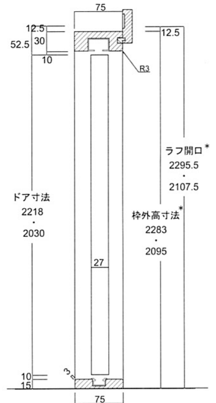
縦断面図
