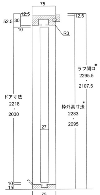
縦断面図
