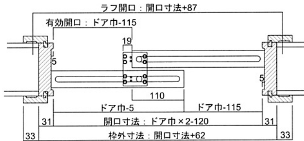
引き違い横断面図
