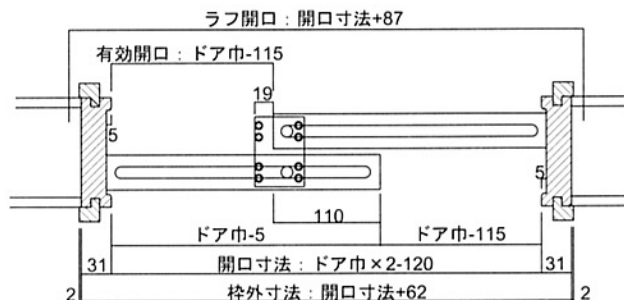
引き違い横断面図
