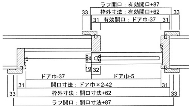
引き違い横断面図
