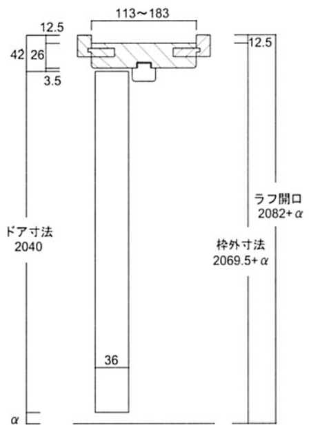
縦断面図
