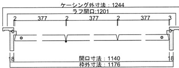
4枚横断面図
