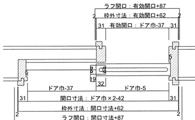
片引き横断面図
