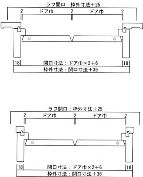
横断面図
