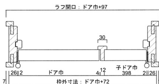
横断面図(親子ドア)
