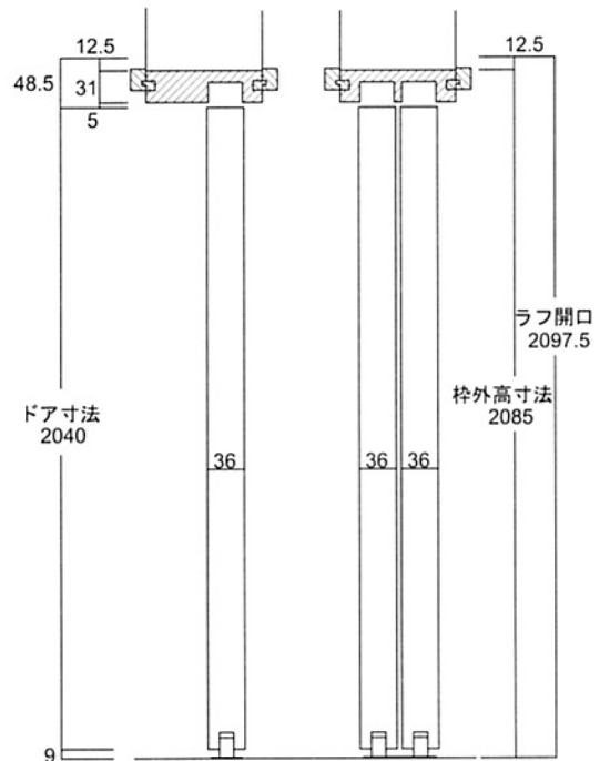
縦断面図
