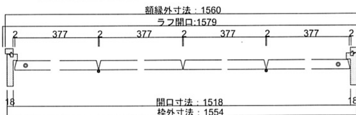
4枚横断面図
