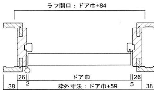
横断面図
