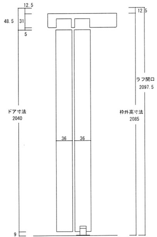
縦断面図
