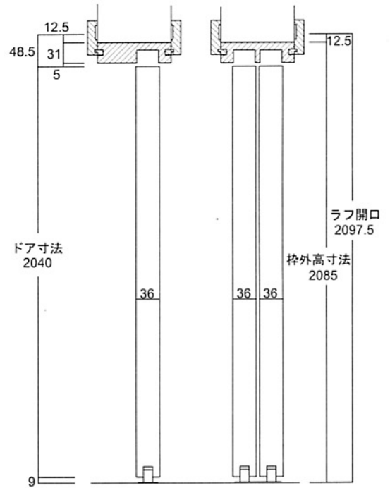
縦断面図
