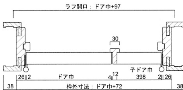
横断面図(親子ドア)
