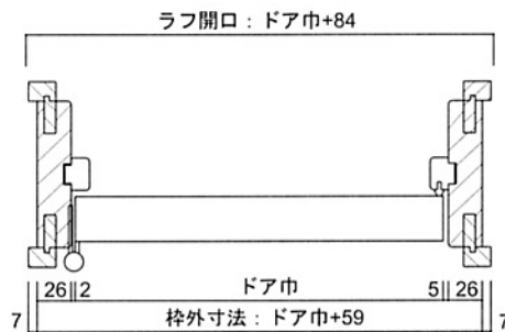
横断面図
