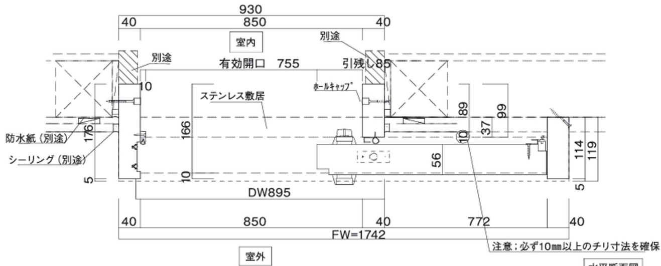
水平断面図
