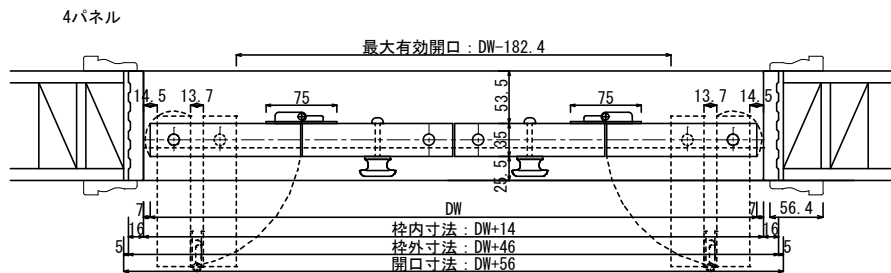
ヘム折戸 標準枠 ※ヘム枠のみ
