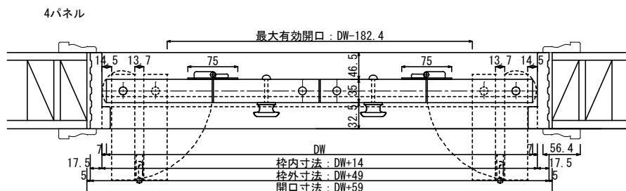
ヘム折戸 三方L型枠 ※ヘム枠のみ
