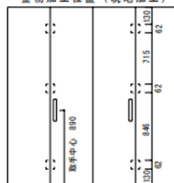
金物加工位置（現地加工）
