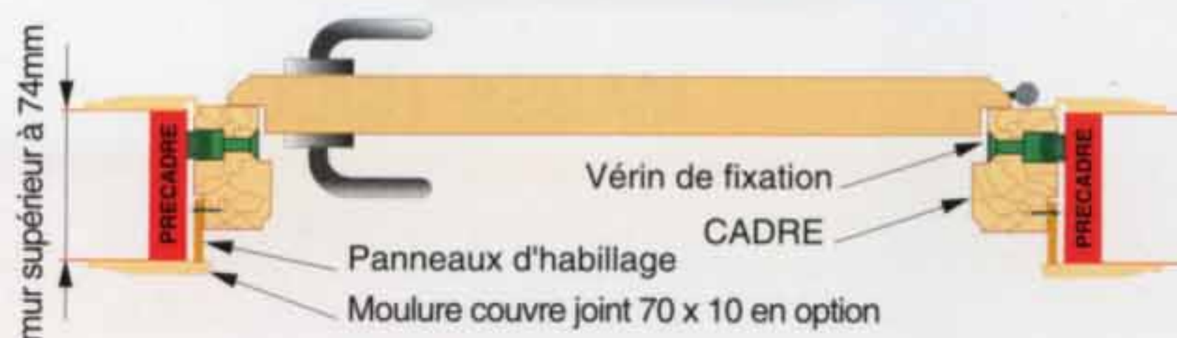
COUPE BP mur > 74 mm
