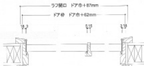
横断面図
