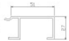
ウェザーストリップ
