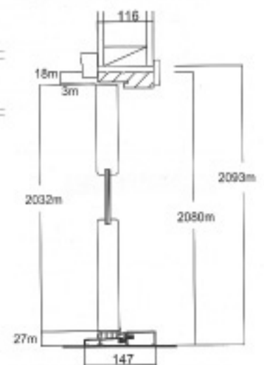
縦断面図
