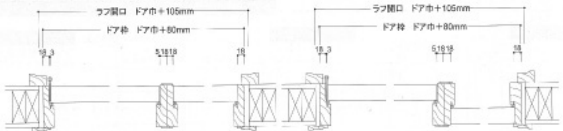
親子ドア(子ドアFIX)Dタイプ
