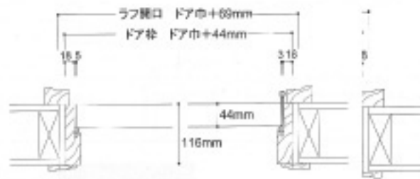
横断面図
