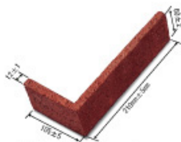
薄レンガIM12RDコーナー ¥450/個 [9012] 約210×約60×約105×約12mm 包装: 30個/ダンボール
